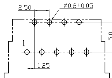
正针 PCB 寸法 Positive needle PCB layout
