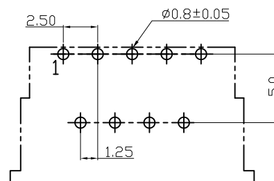
反针 PCB 寸法 Versa needle PCB layout
